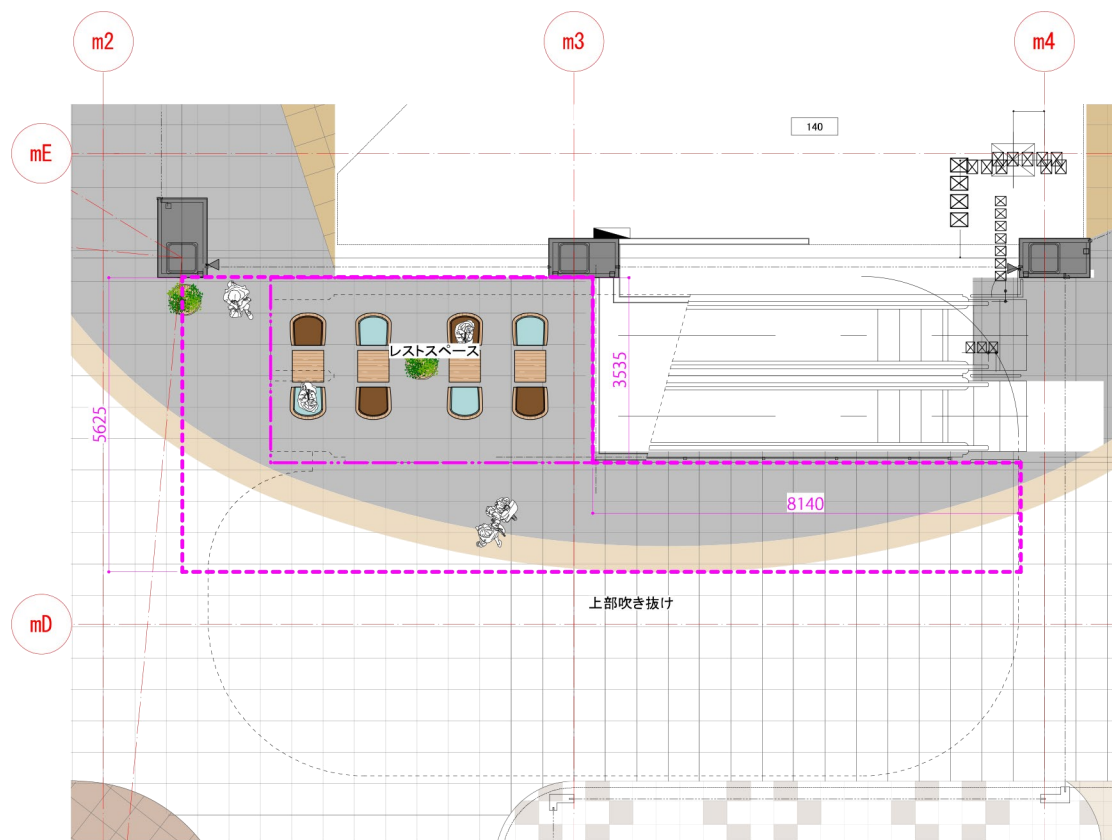
平面図 S=1/100
